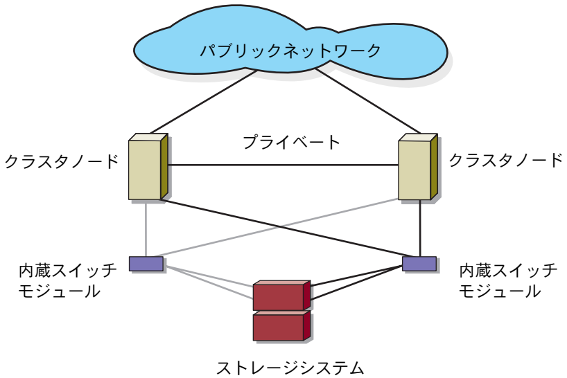
図 1-4. 内蔵パススルーモジュールを使用して外付け SAN に接続したネットワーク接続のクラスタ
