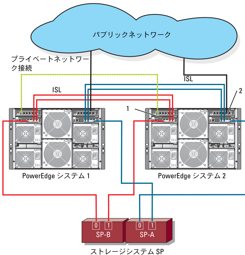
図 2-6. PowerEdge サーバーエンクロージャ 2 台とストレージシステム 1 台を使用したクラスタ構成
