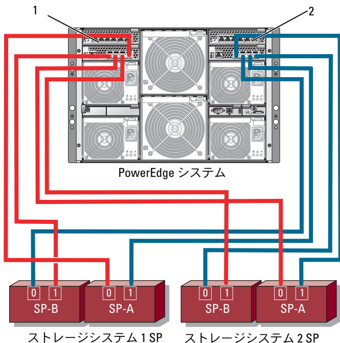
図 2-4. PowerEdge 1855/1955 サーバーエンクロージャ 1 台とストレージシステム 2 台のケーブル接続
