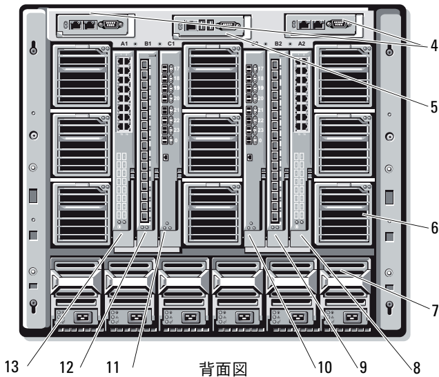
背面図
