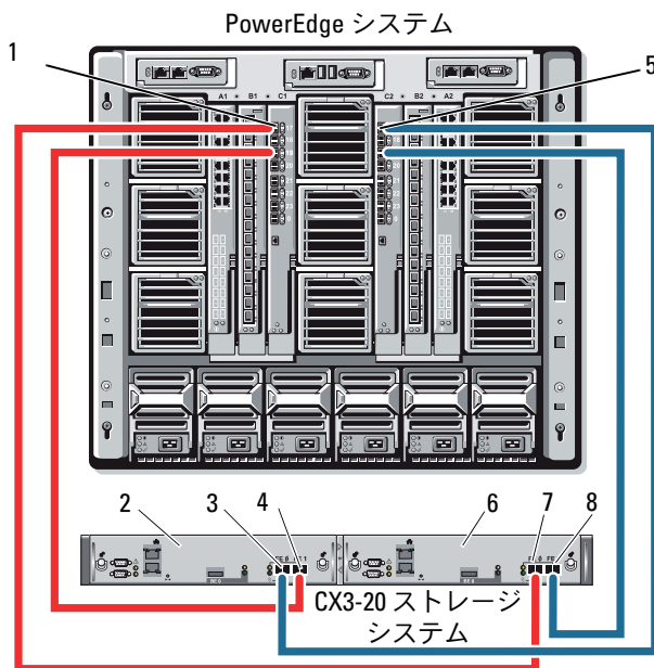
図 2-3. PowerEdge M1000e サーバーエンクロージャ 1 台と CX3-20 ストレージ ロセッサエンクロージャ (SPE) のケーブル接続
