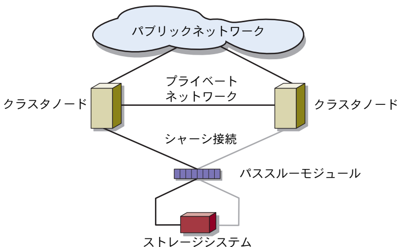
図 1-3. 直接接続クラスタ
