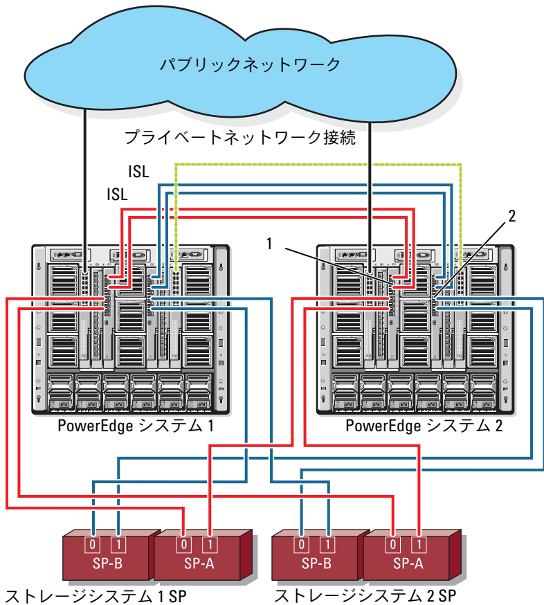
図 2-7. PowerEdge サーバーエンクロージャ 2 台とストレージシステム 2 台の接続
