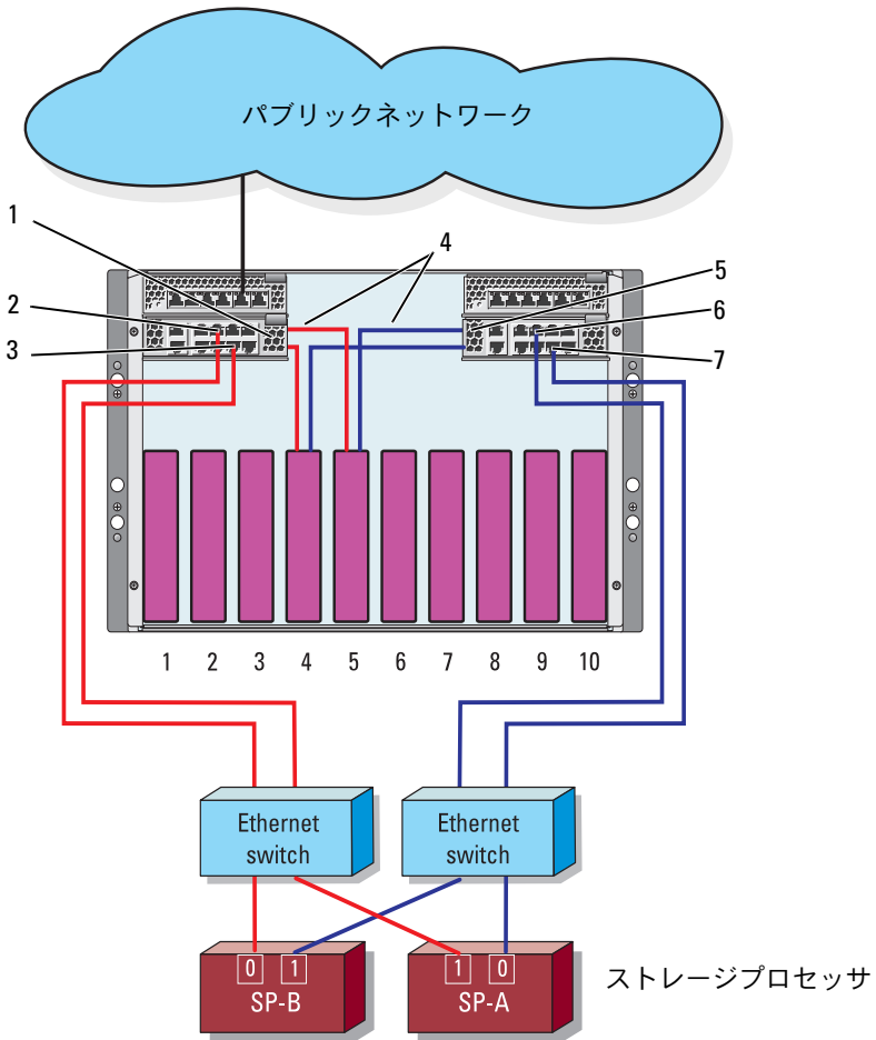
図 2-8. 内蔵イーサネットパススルーモジュールを使用した外付けネットワーク接続の iSCSI クラスタ
