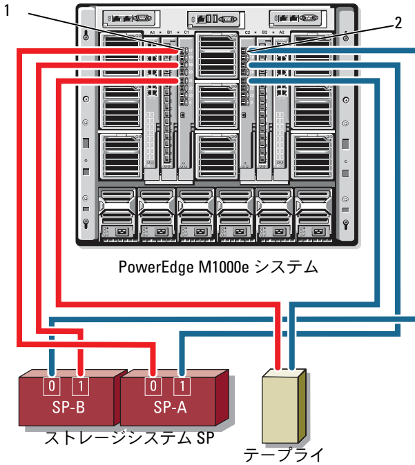
図 2-5. ストレージシステムとテープライブラリのケーブル接続
