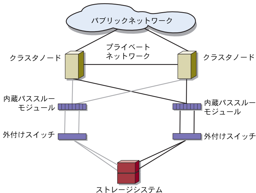
図 1-5. 内蔵スイッチモジュールを使用して外付け SAN に接続したネットワーク接続のクラスタ
