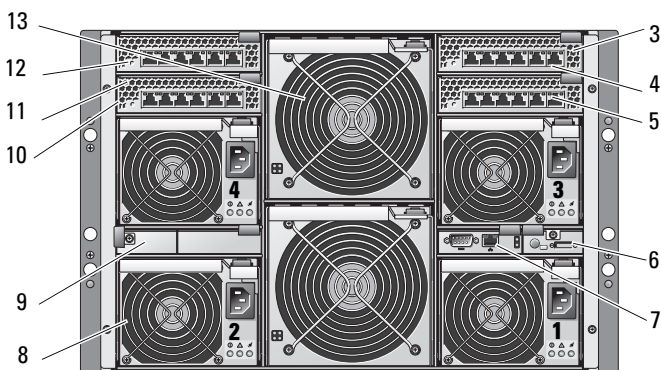
背面図
