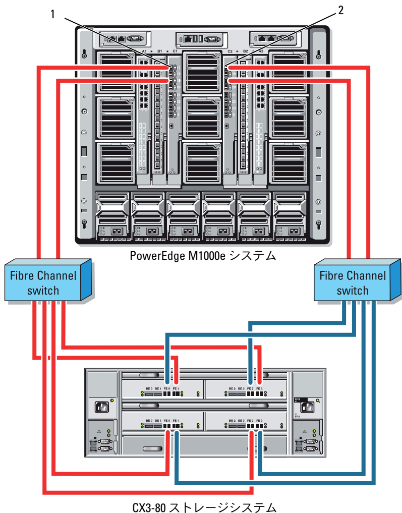
図 2-9. 内蔵ファイバーチャンネルスイッチモジュールを備えた外付けネットワーク接続のクラスタ
