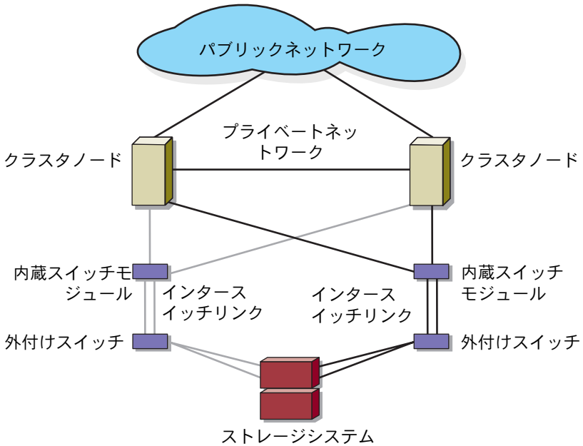
図 1-6. 内蔵パススルーモジュールを使用して外付け SAN に接続したネットワーク接続のクラスタ
